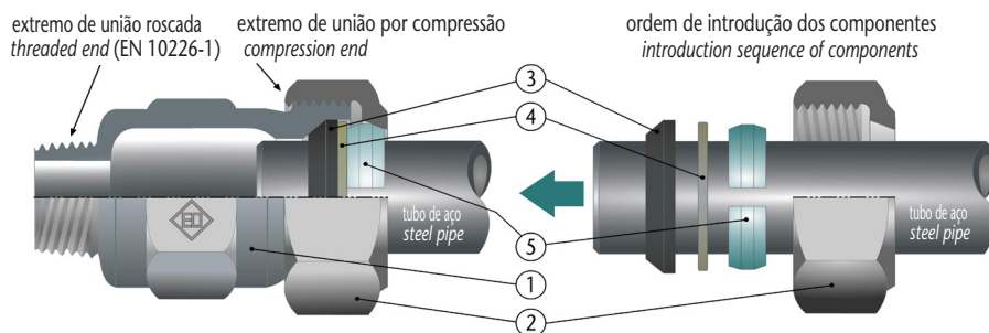
Compressão com porca Nut compression
