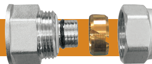
CASQUILHO FÊMEA
