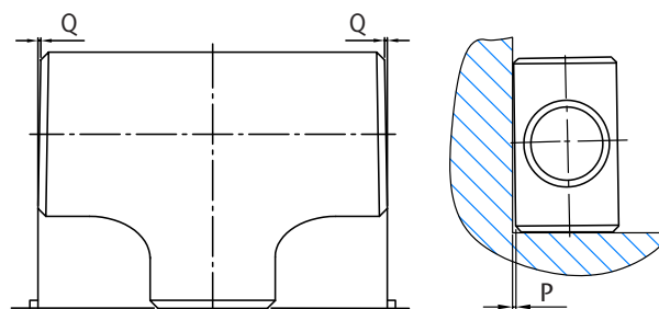
Figura 2 - Forma (exagerada para maior clareza)
