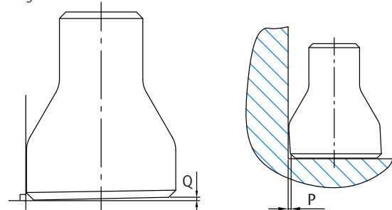
Figura 2 - Forma (exagerada para maior clareza)
