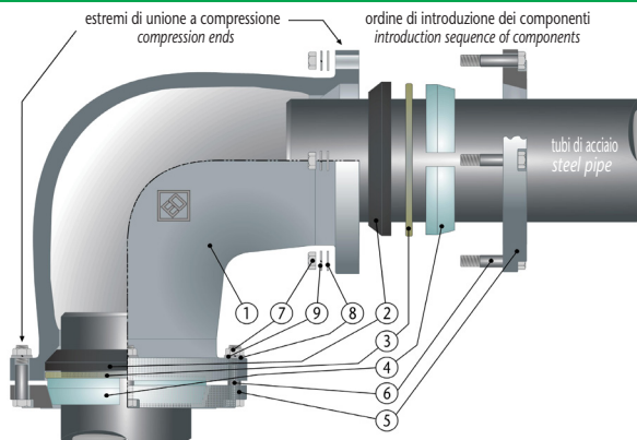
A compressione flangiata Flange compression
