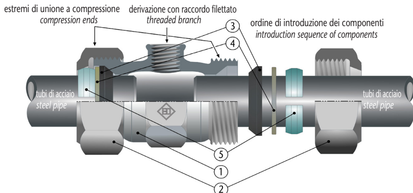
A compressione con dado Nut compression
