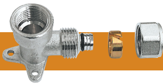
GOMITO FEMMINA CON PIASTRA
