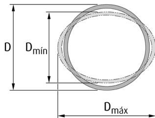
Figura 1 - Ovalità (esagerata per chiarezza) Figure 1 - Ovality (exaggerated for clarity)
