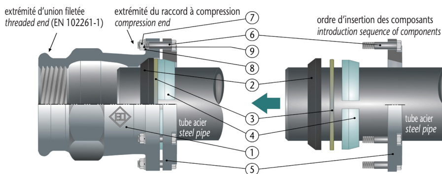
Compression avec bride Flange compression
