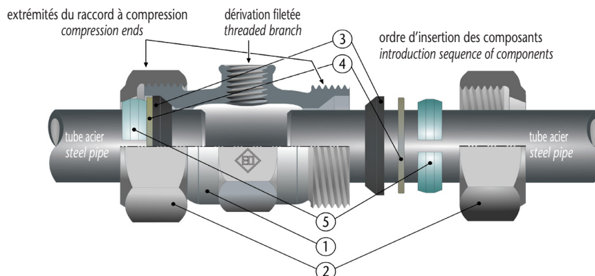
Compression avec écrou Nut compression
