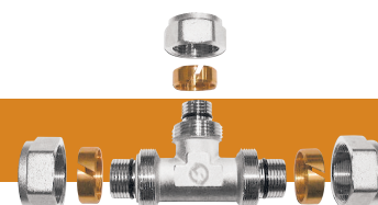
TÉ
