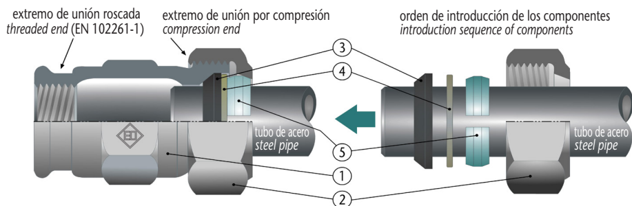
Compresión con tuerca Nut compression
