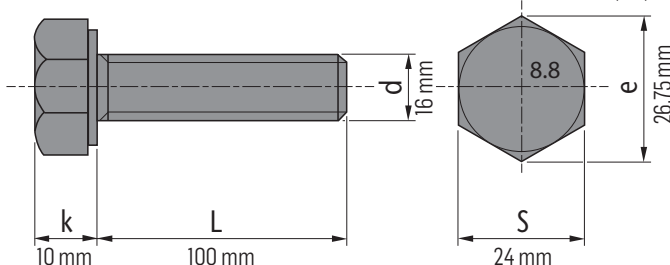
Tornillo de cabeza hexagonal de acero al carbono zincado con rosca total EN ISO 4017 (DIN 933) - Clase 8.8 - Carbon steel hexagonal head bolt with total thread and zinc coated EN ISO 4017 (DIN 933) - Class 8.8
