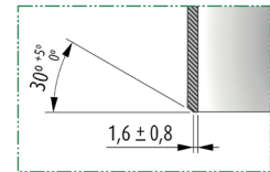
Chafilán del extremo End chamfer
