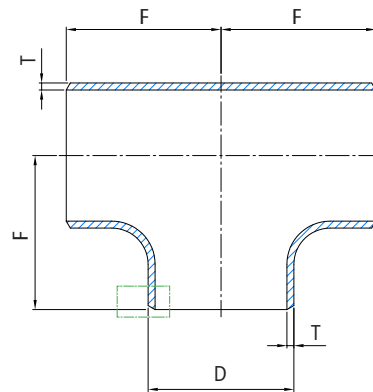
Chafilán del extremo End chamfer
