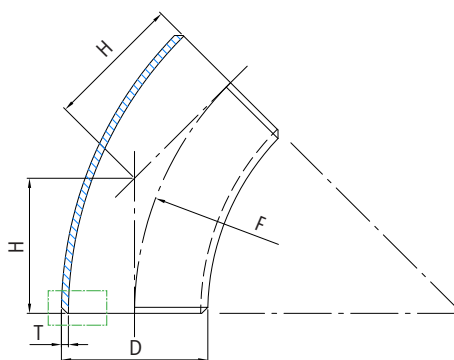
Chafilán del extremo End chamfer
