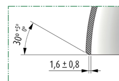
Chablán del extremo End chamfer
