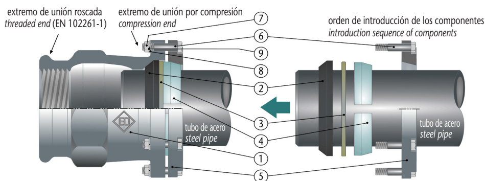
Compresión con brida Flange compression
