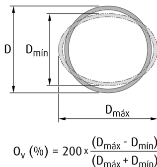
Figura 1 - Ovalidad (exagerada para mayor claridad)
