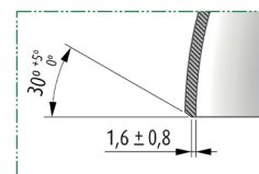
Chablán del extremo End chamfer
